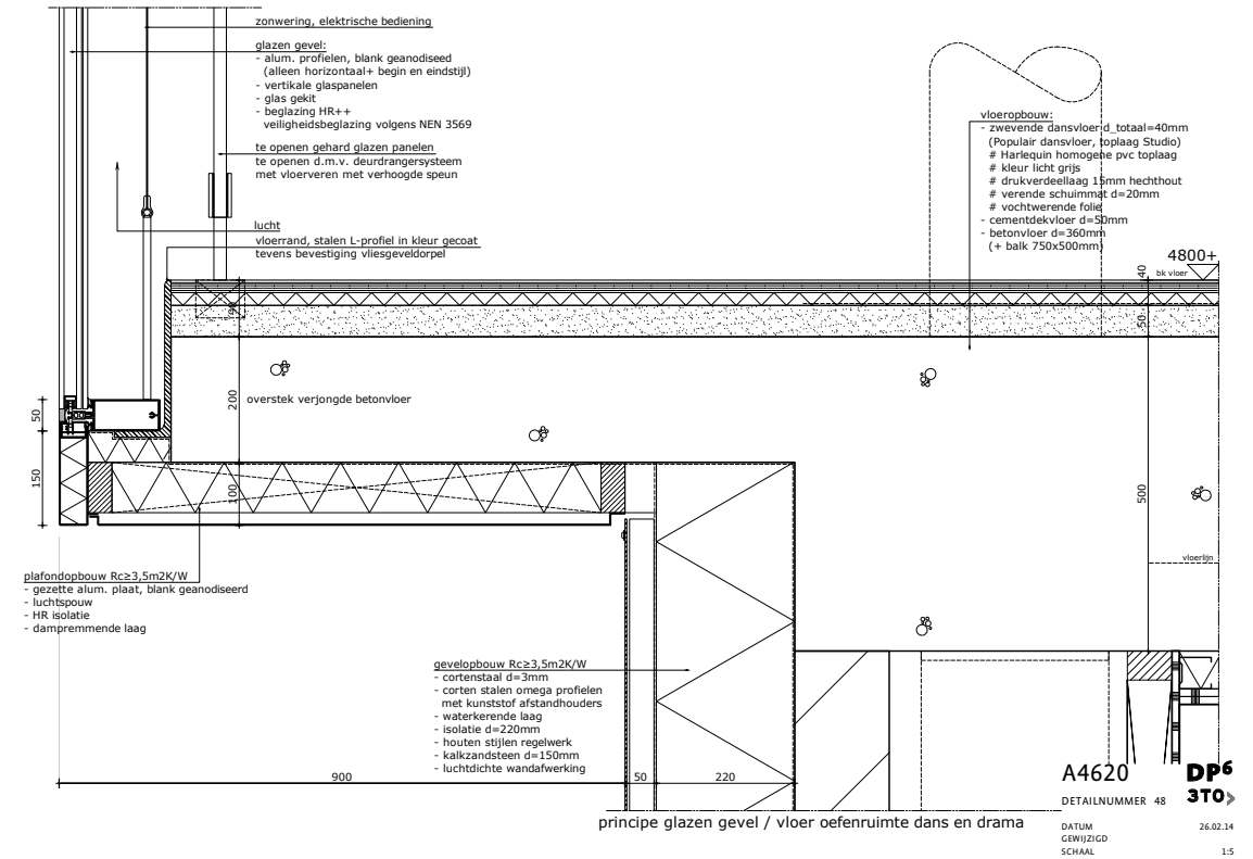
detail 'glazen box' voorgevel
